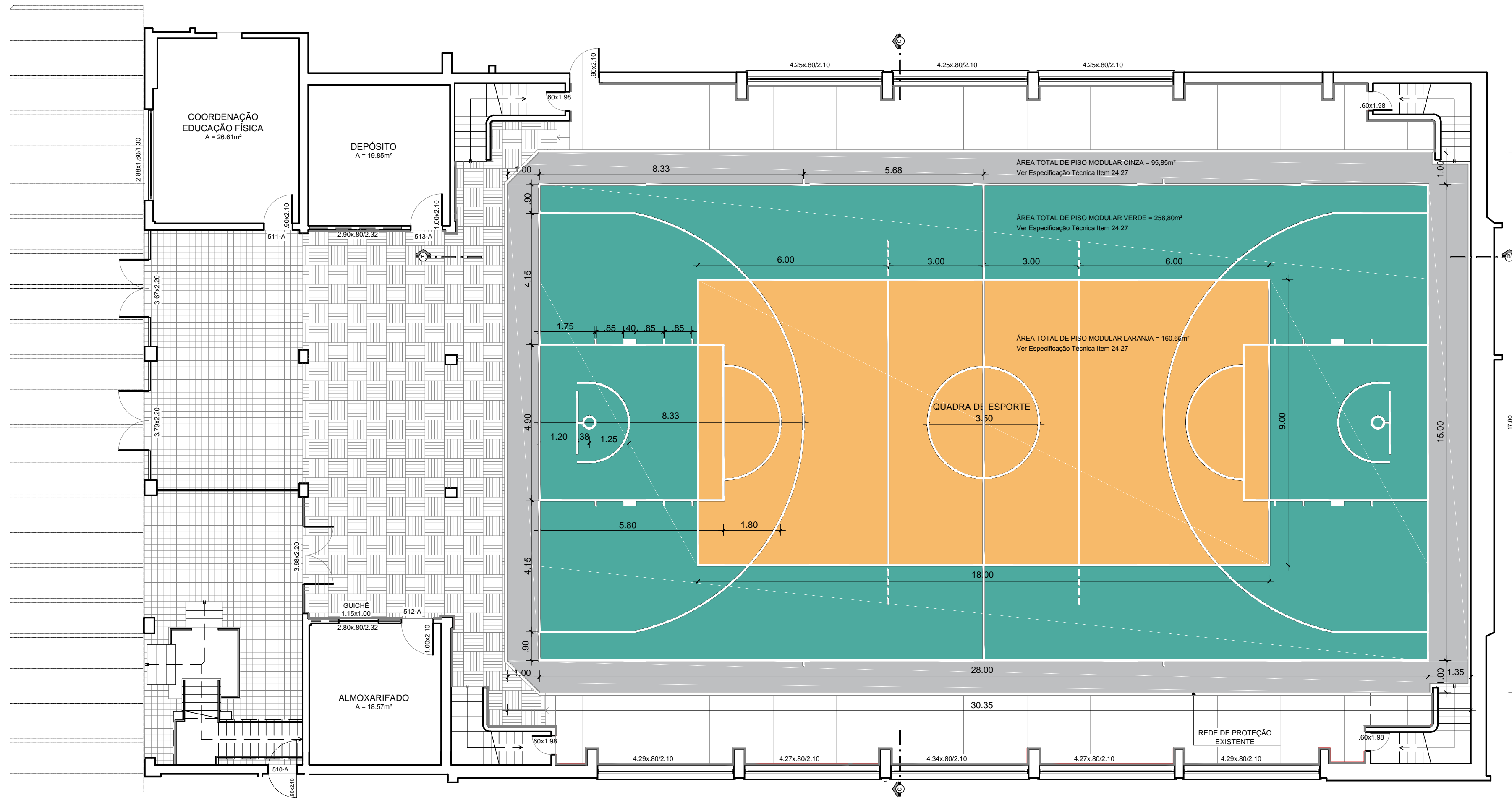
01 PLANTA BAIXA DE PAGINAÇÃO DE PISO ESC: 1/100
